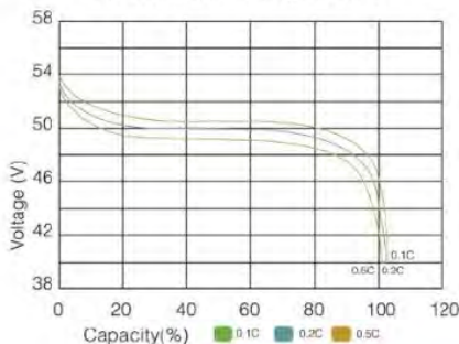
Curva de descarga a 25°C
