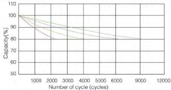
Retención de Capacidad y Ciclos de Vida a distintos DoD a 25°C
